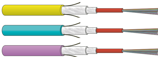
FO Indoor ZGGFR / J-B(ZN)BH
